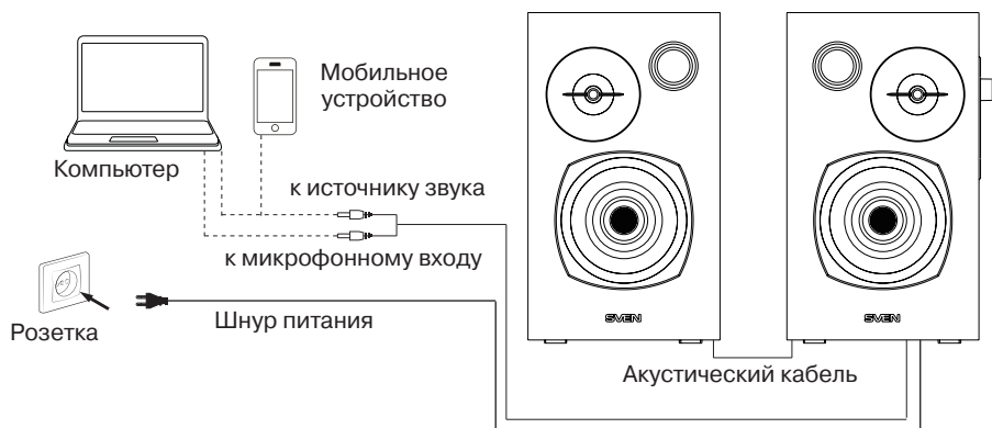
Рис. 2. Схема подключения
