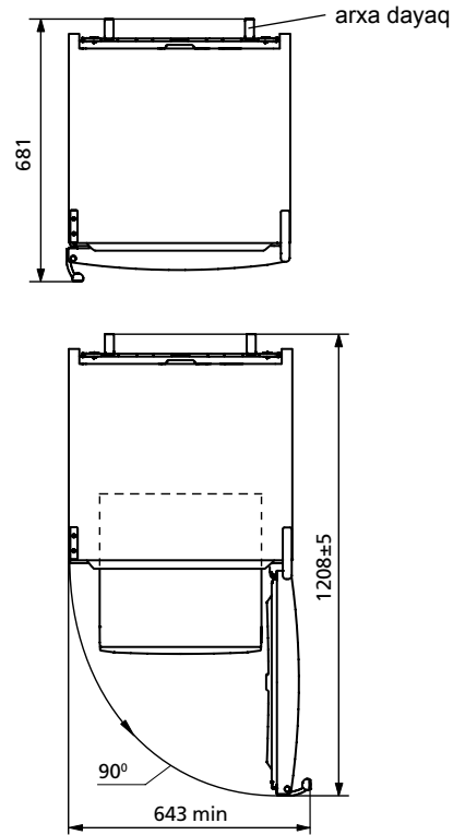
Rəsim 2 – Soyuducu (üstədən görünüşü) bölümünün qapısı
